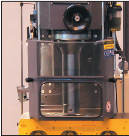
Proteção contra cavacos Protección contra virutas
