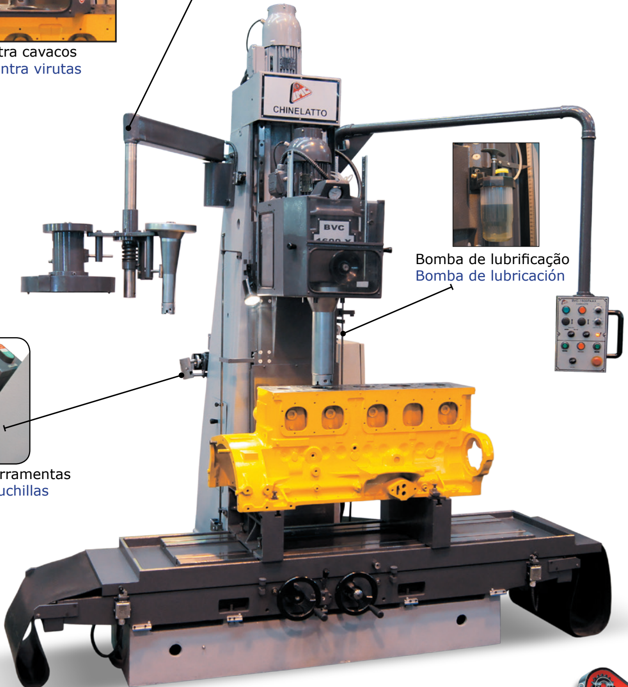
Braço móvel porta-ferramentas Braço móvel porta herramientas
