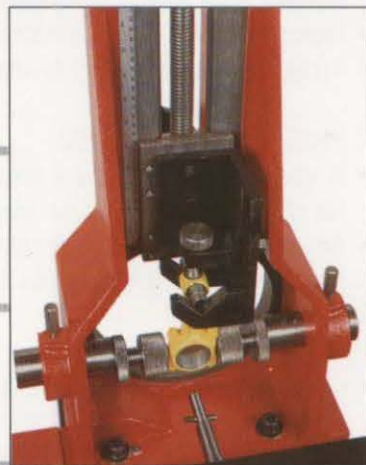
DISPOSITIVO TIPO MESA P/ FIXAÇÃO DE BIELAS PEQUENAS
