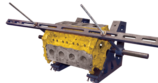
Dispositivo DB-30º/45º p/blocos em "V" Dispositivo DB-30º/45º p/bloques en "V" DB-30º/45º Cradle for "V" blocks
